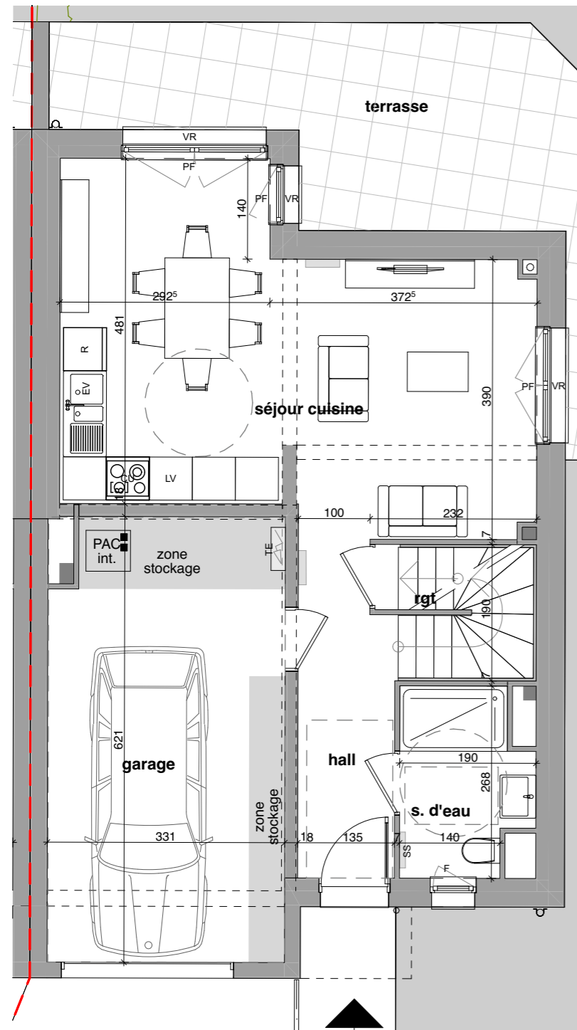
Plan RDC :
