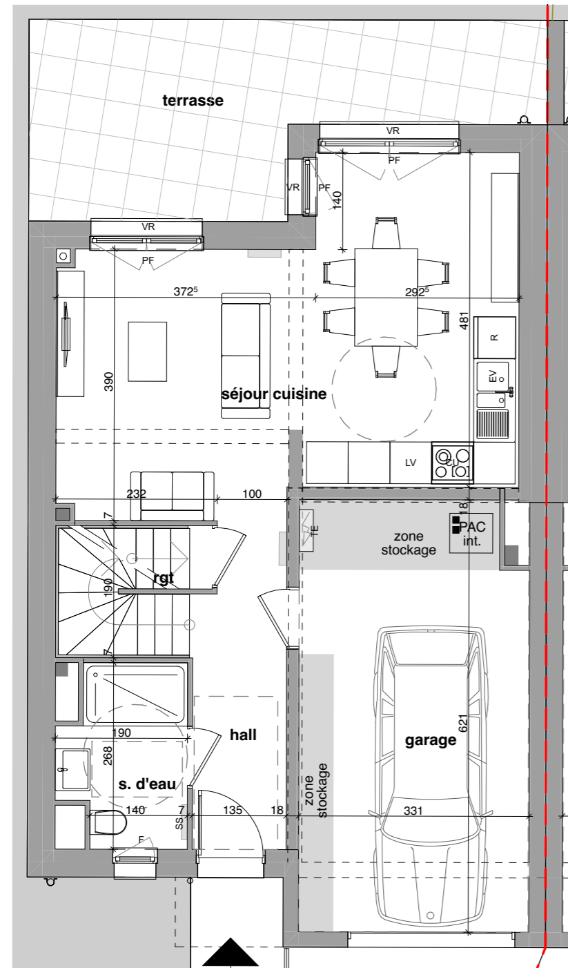
Plan RDC :
