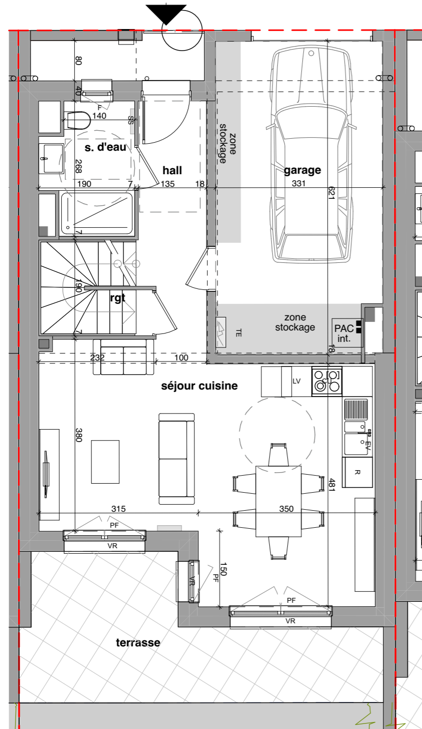
Plan RDC :
