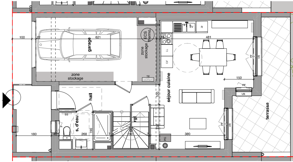
Plan RDC :
