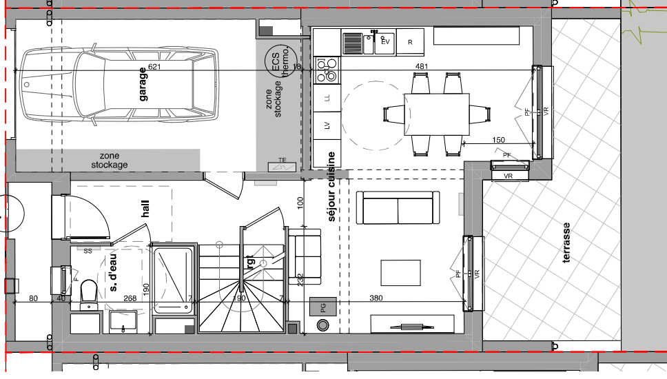
Plan RDC :
