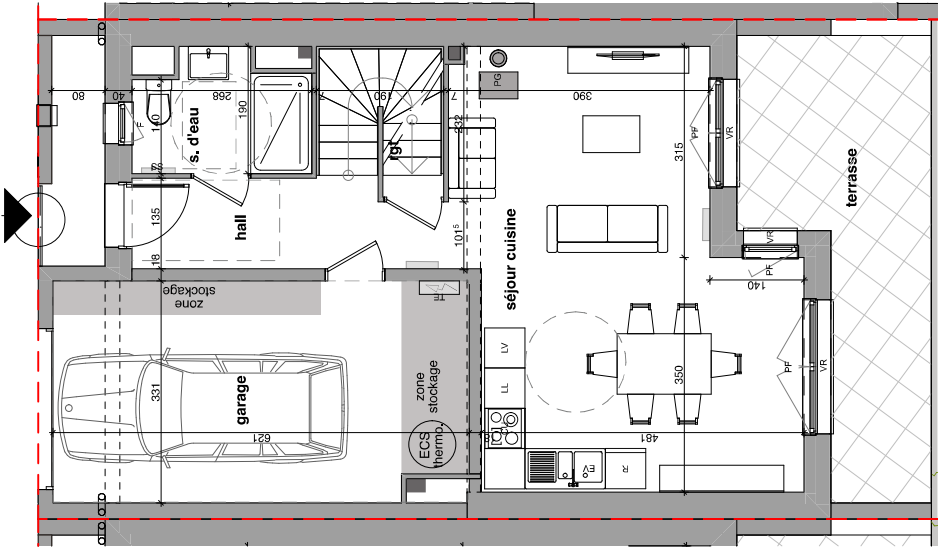
Plan RDC :
