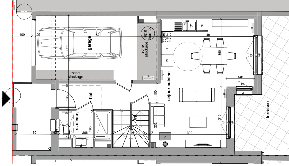
Plan RDC :
