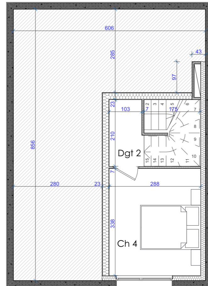
NIVEAU R+2
